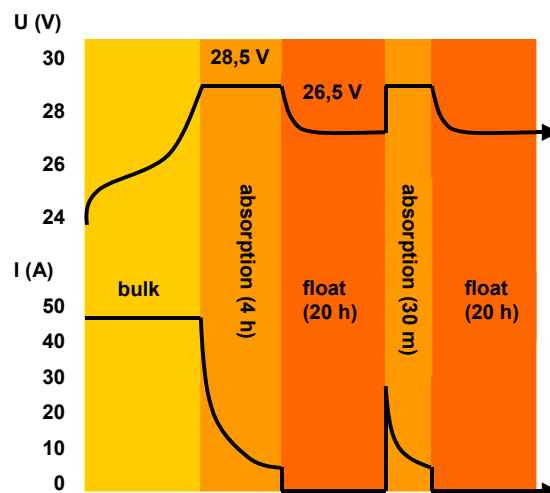
Кривая заряда
